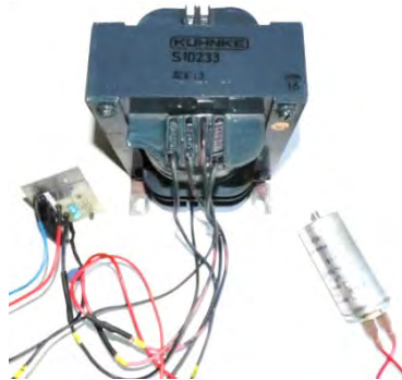
Transformator mit Kondensator KUHNKE S10233 (bh 401127-2000) Kondensator C2200UF/40V (bh401869) Kondensator C47000UF (bh 401869-4740) Transformer and capacitor Bell+Howell PostStar XPO/JPO Art.-Nr.: 8006.01 gebraucht- wie abgebildet Preis pro Stück: 10,00 €
