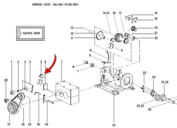
Abb.01, 02, 03 Rillenkugellager DIN 625-634-2 rs1 (bh 413579-0001) Exenterachse D=17 (bh 415480) Klemmring DI=17 H 7 DA=50 (bh 414637-0009) - Ball bearing Bell+Howell CE,CEX,CEXP/XPO/JPO Art.-Nr.: 8338 gebraucht - wie abgebildet Preis pro Stück:
