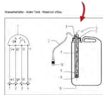
Wasserbehälter - Water Tank - Reservoir d'Eau 1 046316-0002 Anschlußplan Füllstand Wasser-tank 2 430426-109 Unabgeschirmte PVC-St.leitung 8 x 0,25 3 405285 Kabeldurchführung 4 414545-0004 Schlauch Silikon DI = 4 mm 5 218107-01 Sicherungerring DIN 471-26 x 1,2 6 411734 Wasserbehälter 10 l 7 414883-0001 Rohr für Füllstandskontrolle 8 412565-0003 Anschlußstück 9 414292-0001 Füllstandssensor 10 403937-0001 Kupplungsdose 6 polig rund
