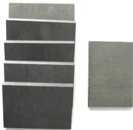
Lamelle Kohleschieber für Rietschle Vakuumpumpe TLV 15 (13)513702 103808919 B 55mm x H 39 mm x 4,5mm Verpackungseinheit 6 Stück Art.-Nr.: 8227 Preis pro Stück:
